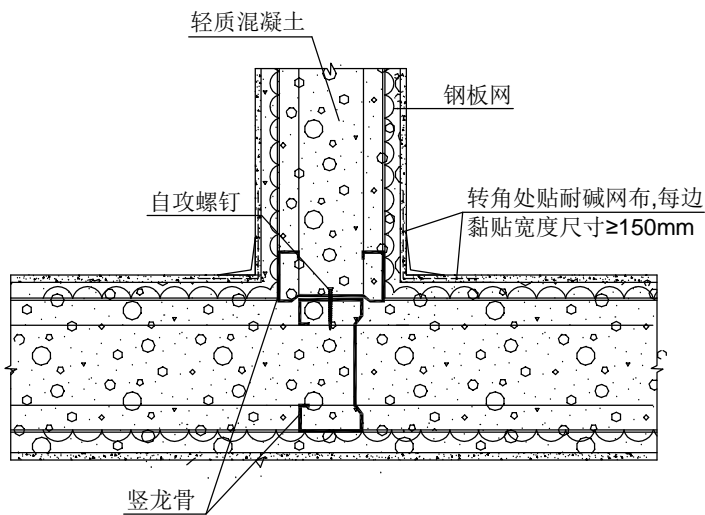
② T型 (2)
