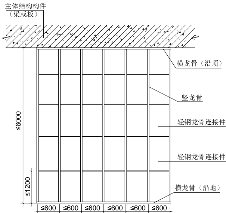
轻钢龙骨墙体骨架布置图 (1)
