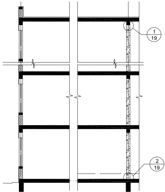
1-1剖面图
