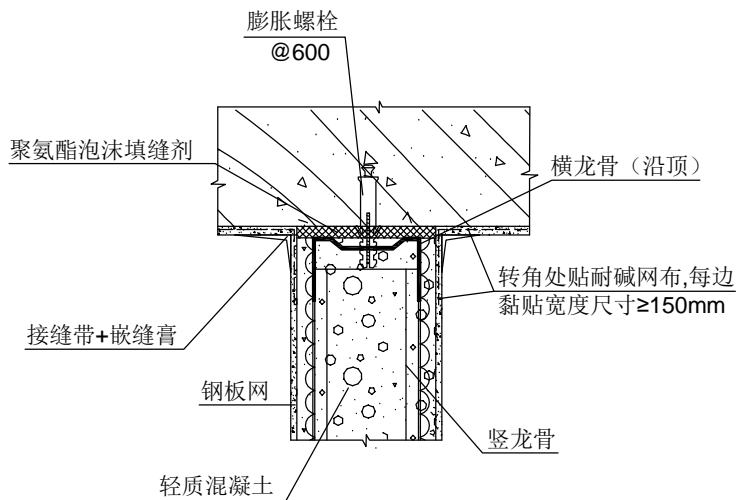
① 与顶棚连接
