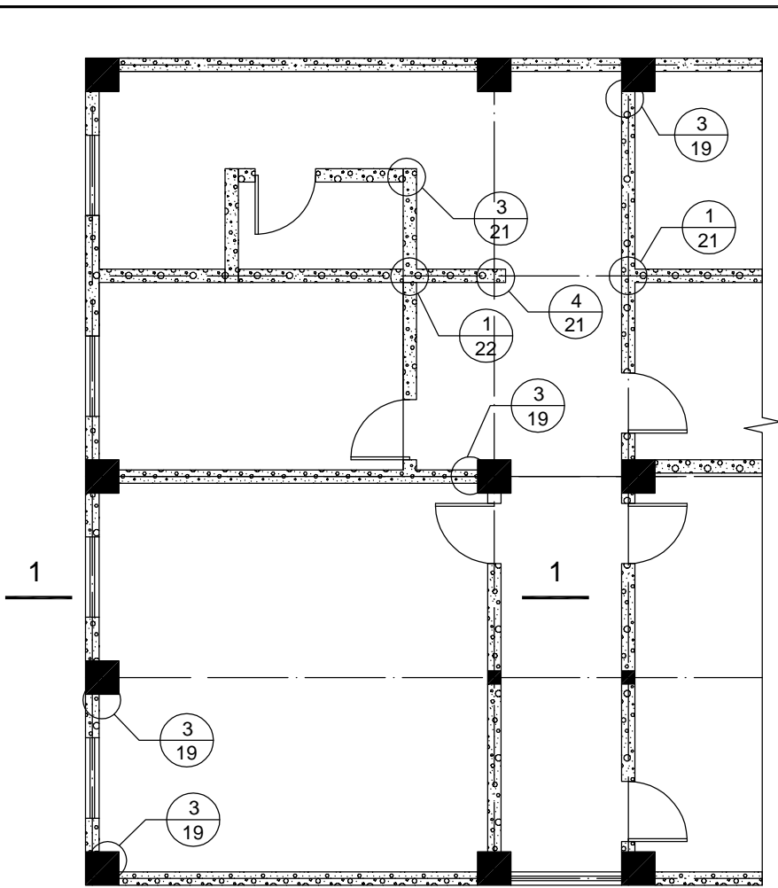
建筑平面图
