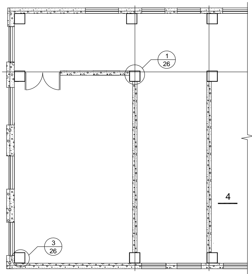
建筑平面图
