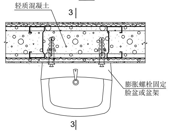
③ 洁具安装
