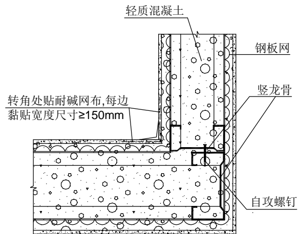
③ L型
