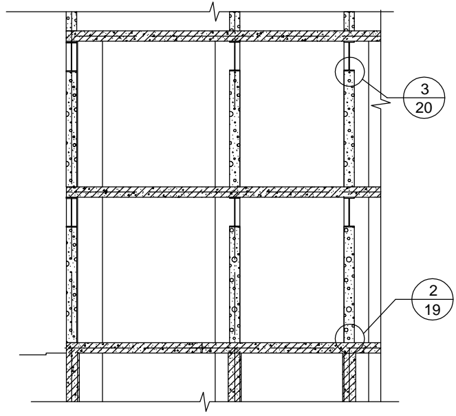
3-3剖面图
