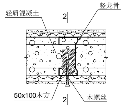
② 竖龙骨吊挂 (吊挂重量25~35kg)
