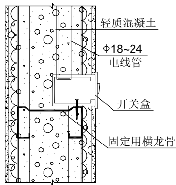
① 开关盒
