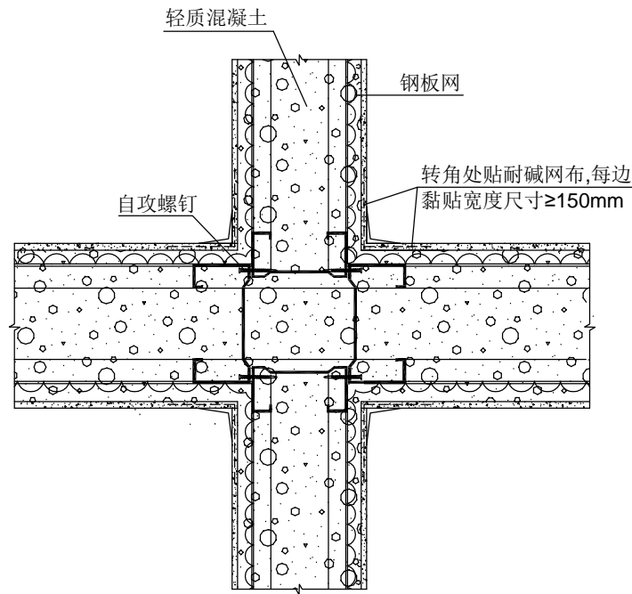
② 十字型 (2)
