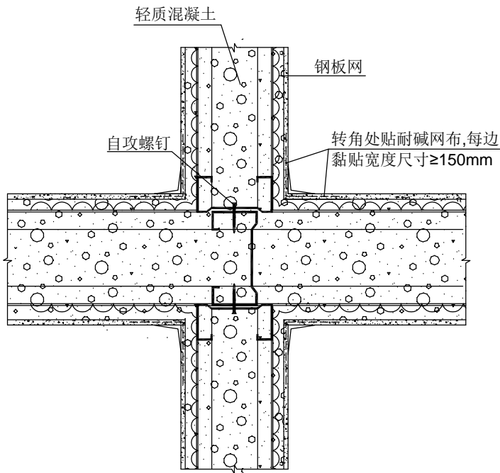
① 十字型 (1)
