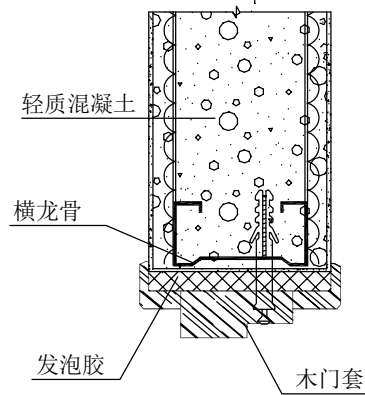
② 木门套
