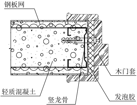
⑤ 木门套
