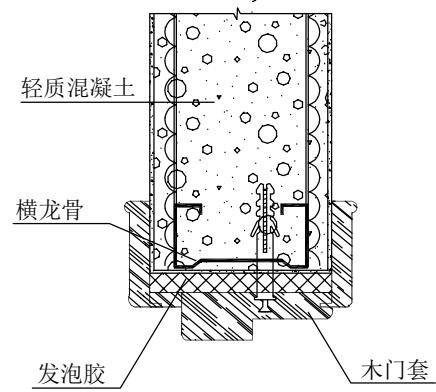
④ 木门套
