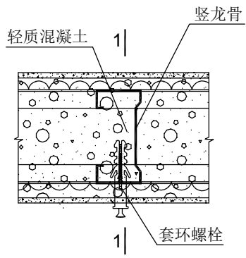
① 竖龙骨吊挂 (吊挂重量25~35kg)
