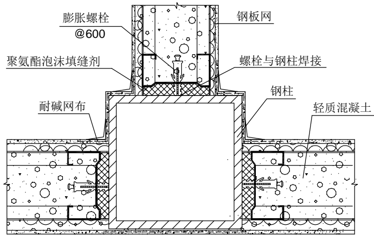
① 复合墙体与钢结构连接 (3) T型
