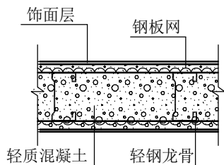
图1 网模轻质混凝土内隔墙体基本构造示意
