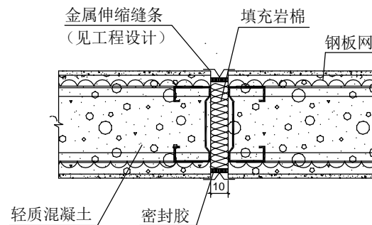
伸缩缝构造
