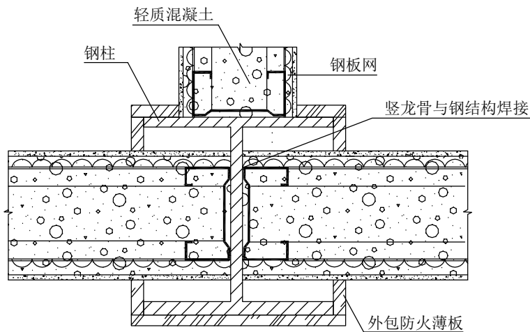
① 复合墙体与钢结构连接 (2) T型
