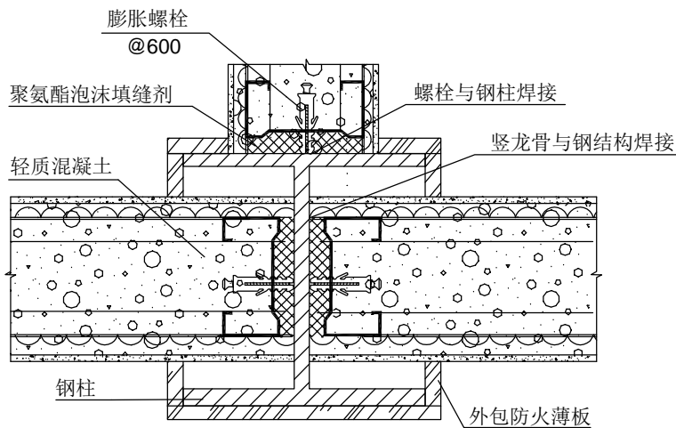
① 复合墙体与钢结构连接 (1) T型
