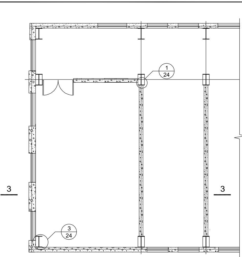
建筑平面图
