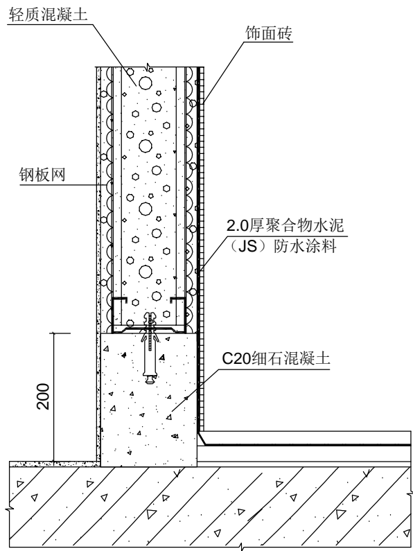
与卫生间楼地面连接
