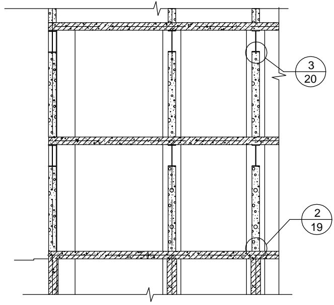
4-4剖面图
