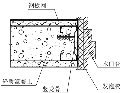
③ 木门套
