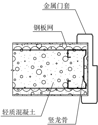
① 金属门套
