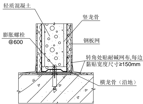
② 与楼地面连接
